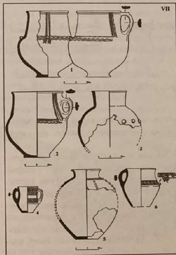
Рис. 6-7. Инвентарь погребения № 1 с каменной насыпью. Керамика
