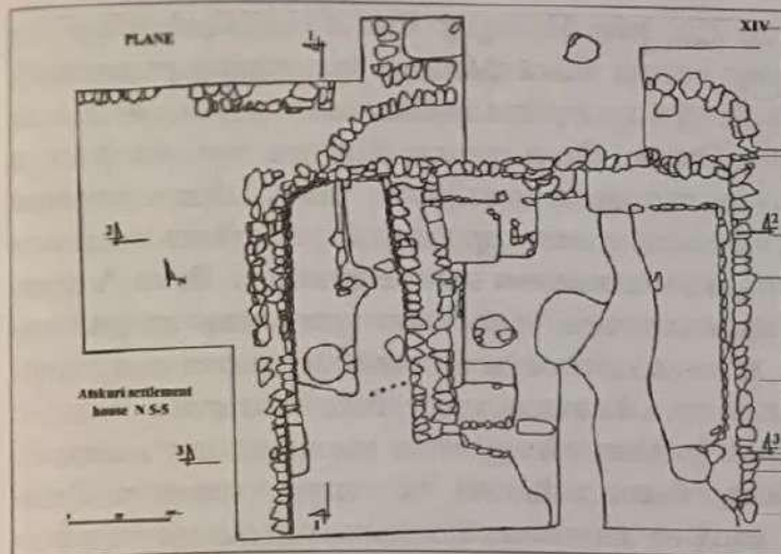
Рис. 14-15. Дом № 5 городища Ацкури. План и разрез
